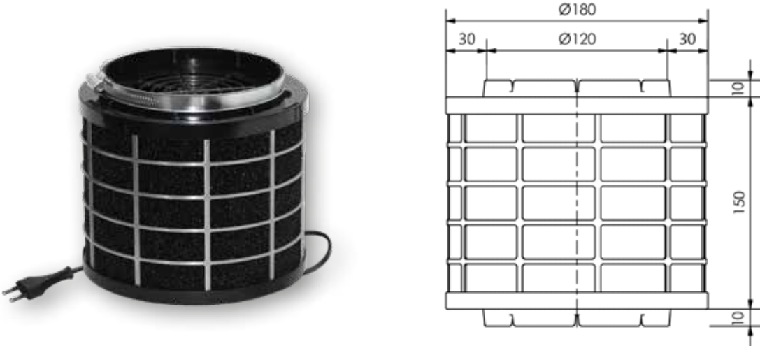
RONDO 400 | MA Ø 120 mm
