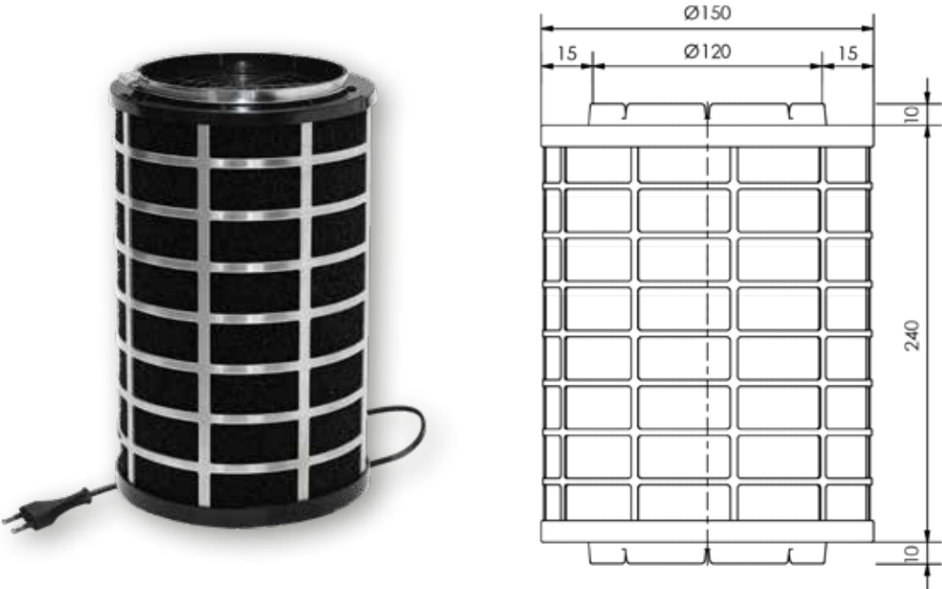
RONDO 650 | MA Ø 120 mm
