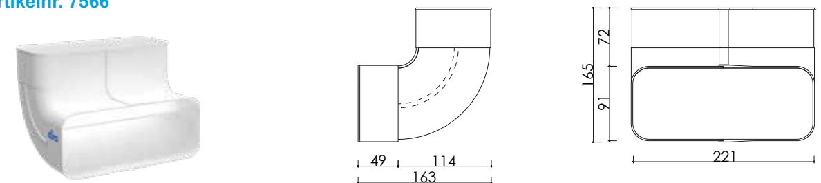
QUADRO bocht verticaal 90° Artikelnr. 7566
