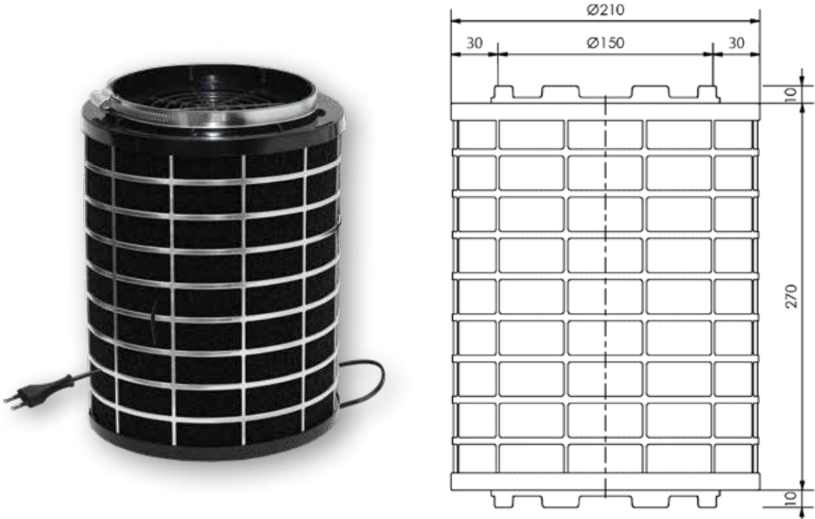
RONDO 1000 | MA Ø 150 mm
