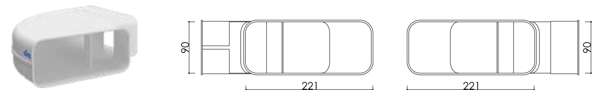
QUADRO bocht horizontaal 90° Artikelnr. 7565
