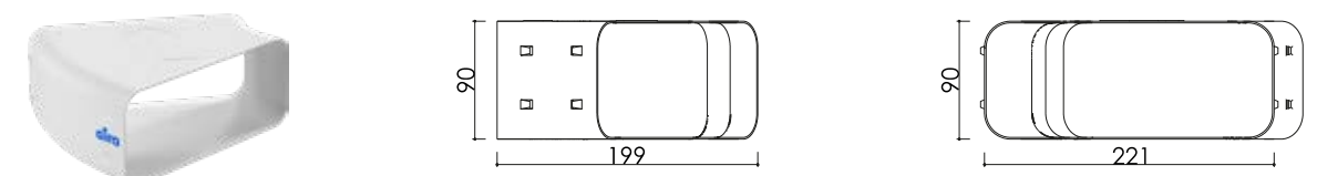
QUADRO bocht horizontaal 30° Artikelnr. 7570
