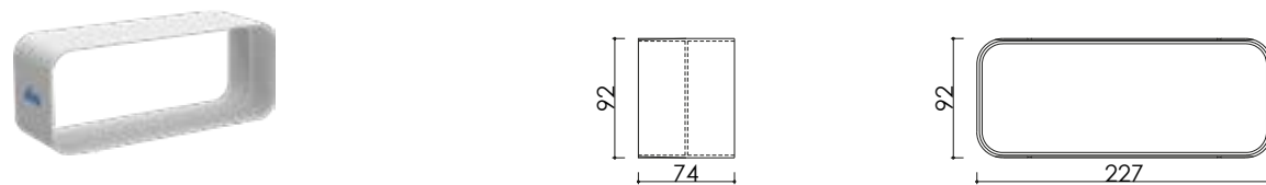
QUADRO mof Artikelnr. 7557
