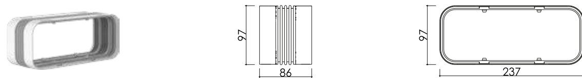
QUADRO universele connector Artikelnr. 7557_Flex
