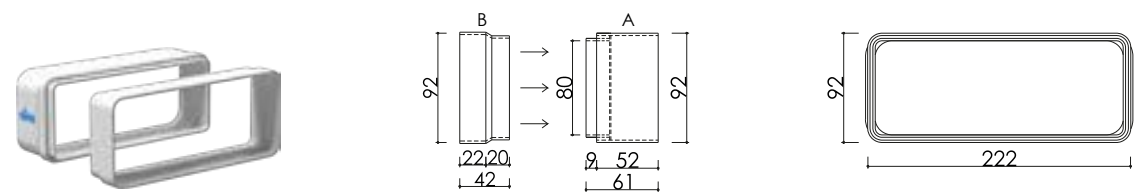
QUADRO Adapter Internationaal Artikelnr. 7569
