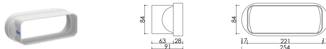
Bora adapter Artikelnr. 7577
