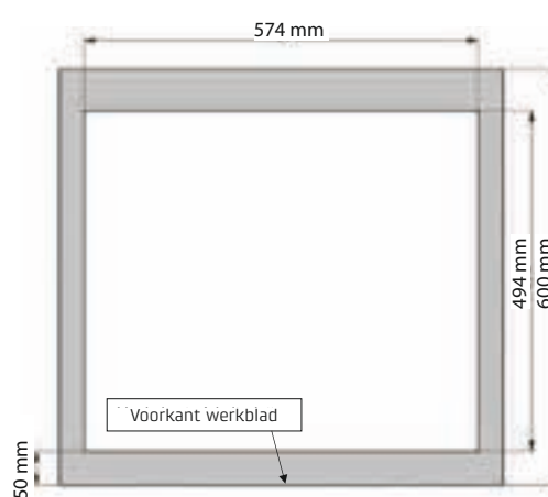
Inbouw montage opbouw
