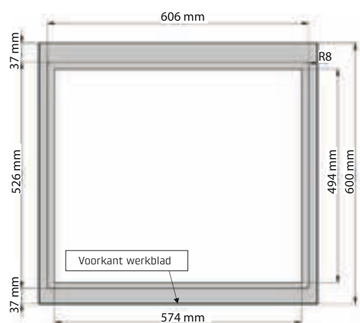
Vlak Inbouw met sponning
