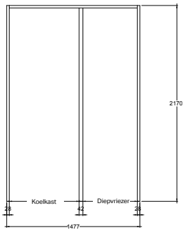
VOORAANZICHT
