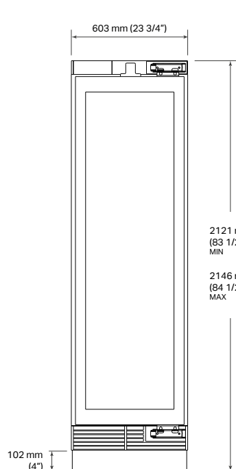
VOORAANZICHT
