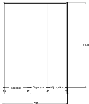
VOORAANZICHT
