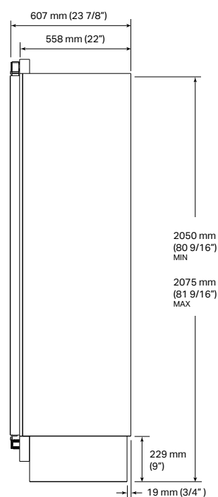
ZIJAANZICHT
