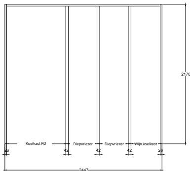
VOORAANZICHT
