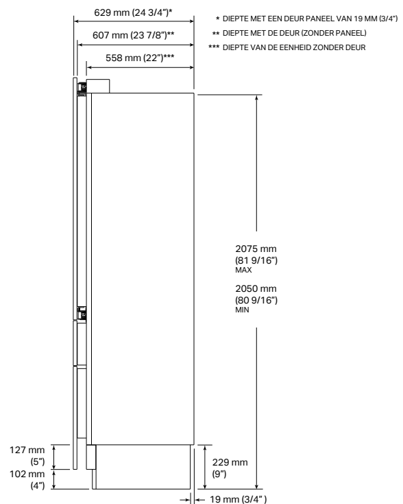
ZIJAANZICHT
