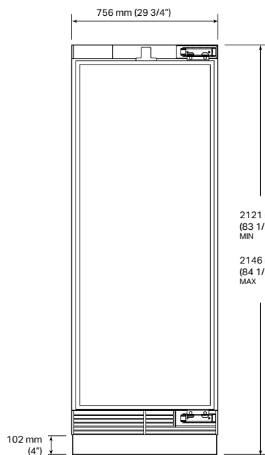
VOORAANZICHT
