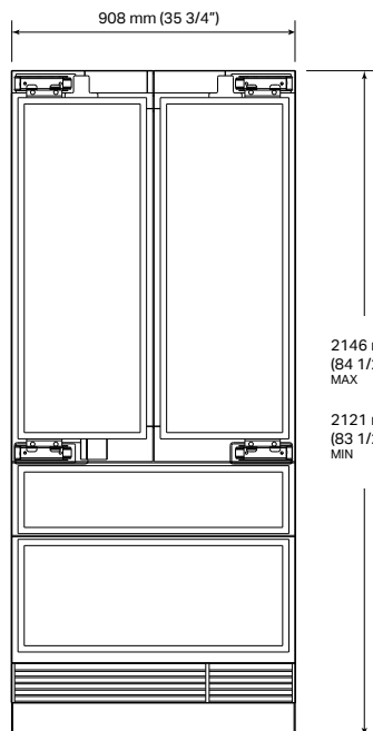
VOORAANZICHT
