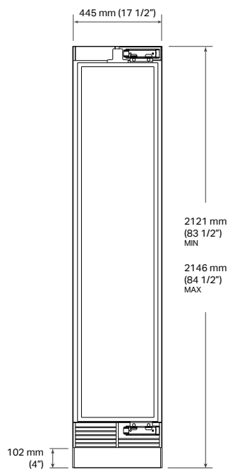
VOORAANZICHT
