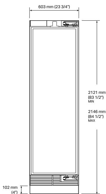
VOORAANZICHT
