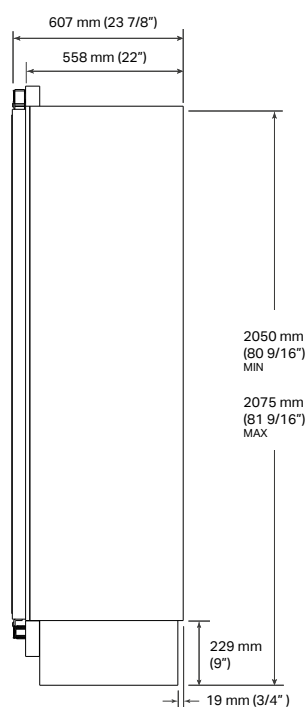
ZIJAANZICHT
