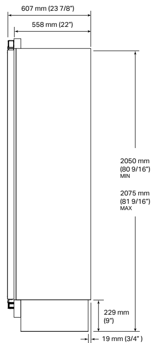
ZIJAANZICHT
