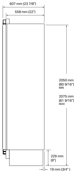
ZIJAANZICHT
