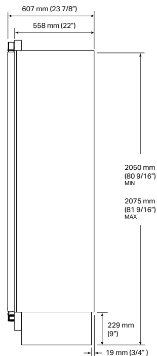
ZIJAANZICHT
